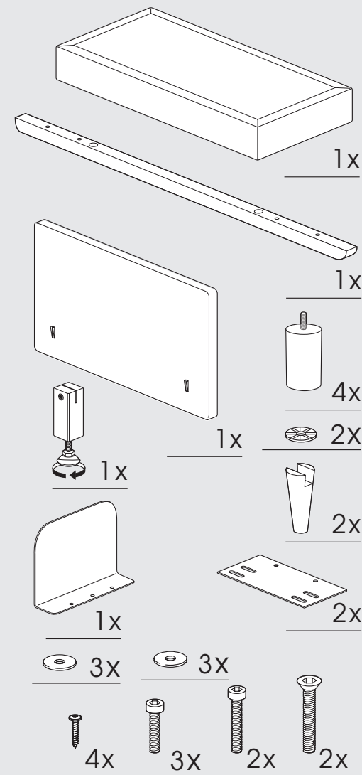
HOLZLEISTE VORNE TRAVERSE EN BOIS, AVANT WOOD BEAM WOODEN FRONT BEAM
